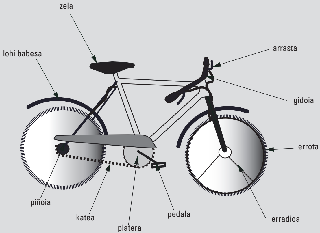
Bizikletaren eskema
